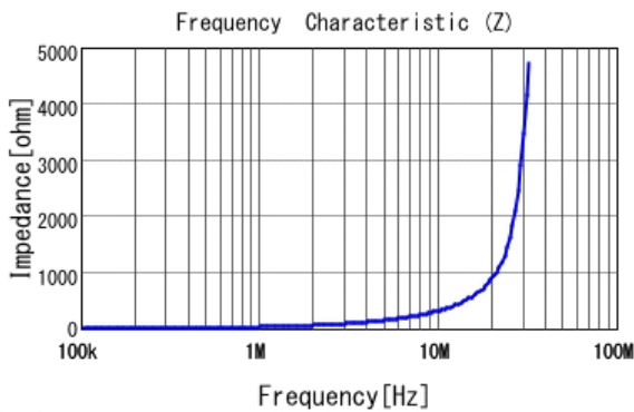
■ 1269AS-H-4R7M |Z|
