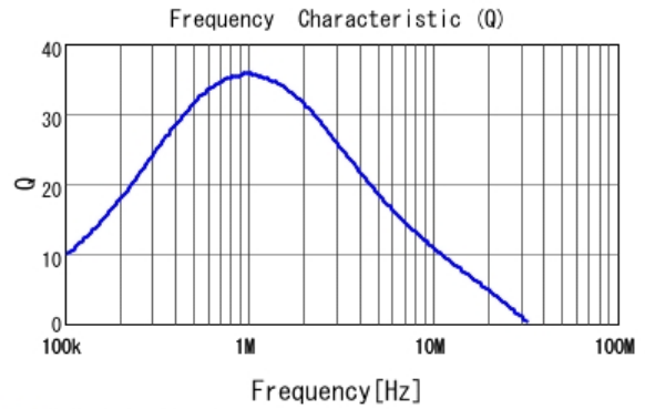
■ 1269AS-H-4R7M Q
