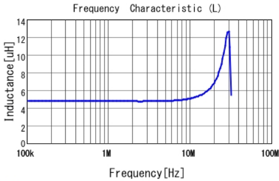
■ 1269AS-H-4R7M L
